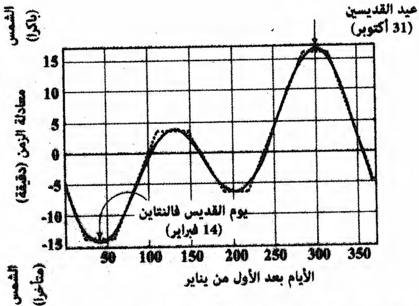
الشكل (90): معادلة الزمن والتقريب منقط فوقها.
